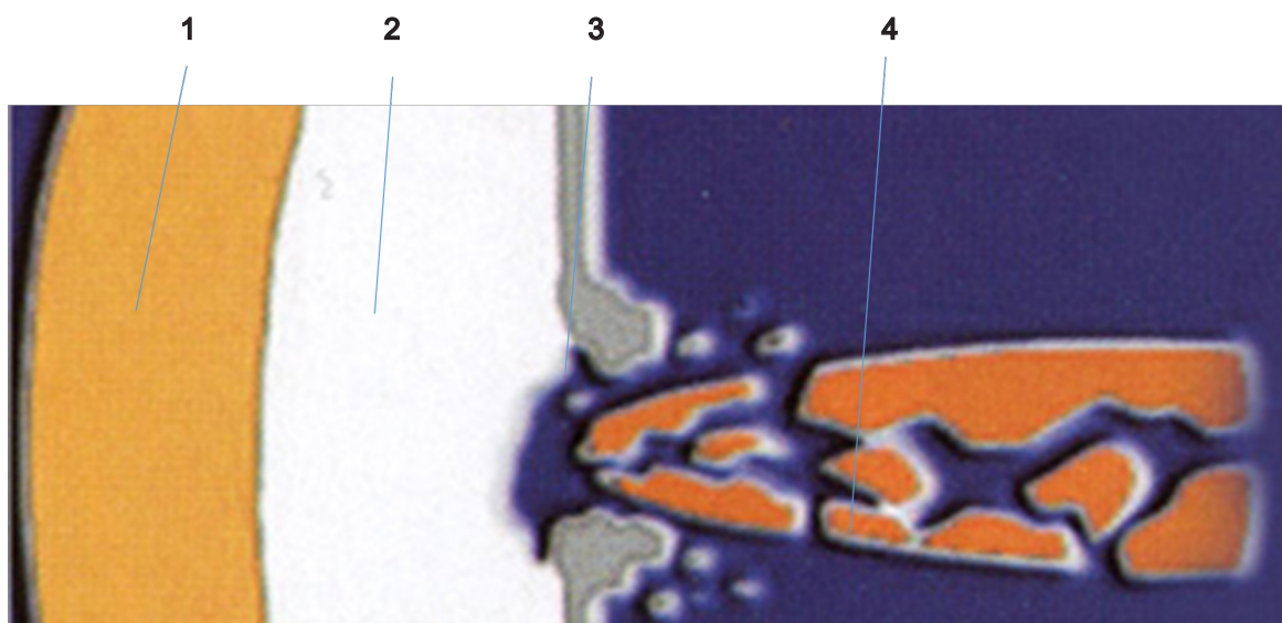
სურ. 1. მრავალშრიანი საჯავშნე სისტემის დაზიანების სქემა; 1-ჭურვი, 2- ბოჭკოვანი შრე, 3- კერამიკა, 4- კიდურა დამცავი ელემენტი.
